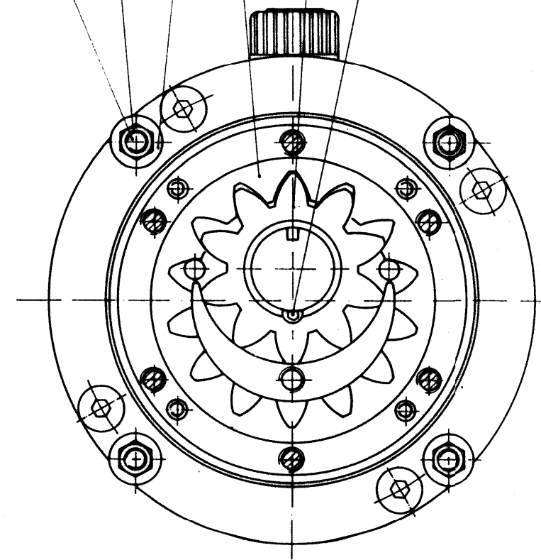
SNITT SECTION A-A
